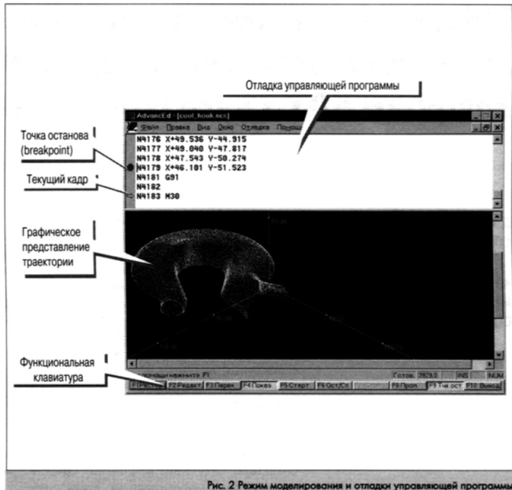
Рис. 2 Режим моделирования и отладки управляющей программы
